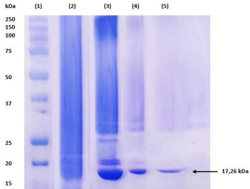
Gambar 2. Hasil elektroforesis SDS-PAGE protein Ngb
